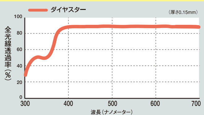
●光線透過特性
