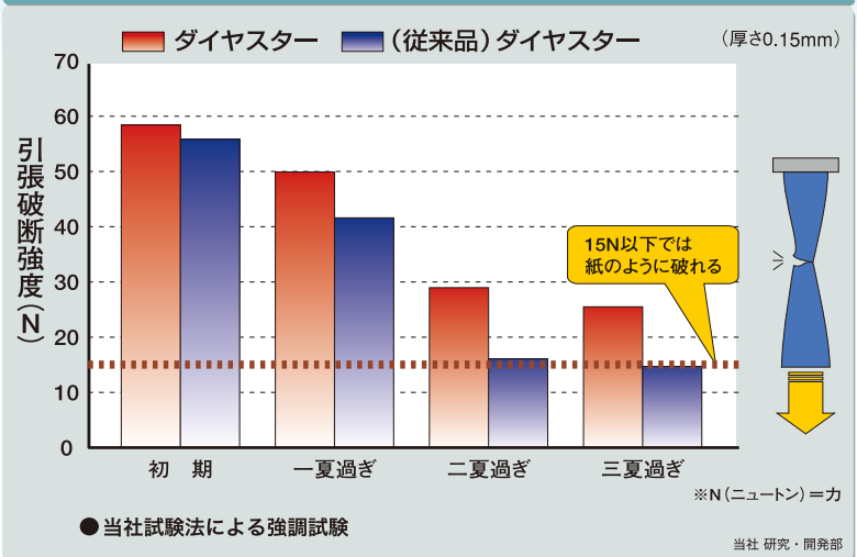
引張強度比較
