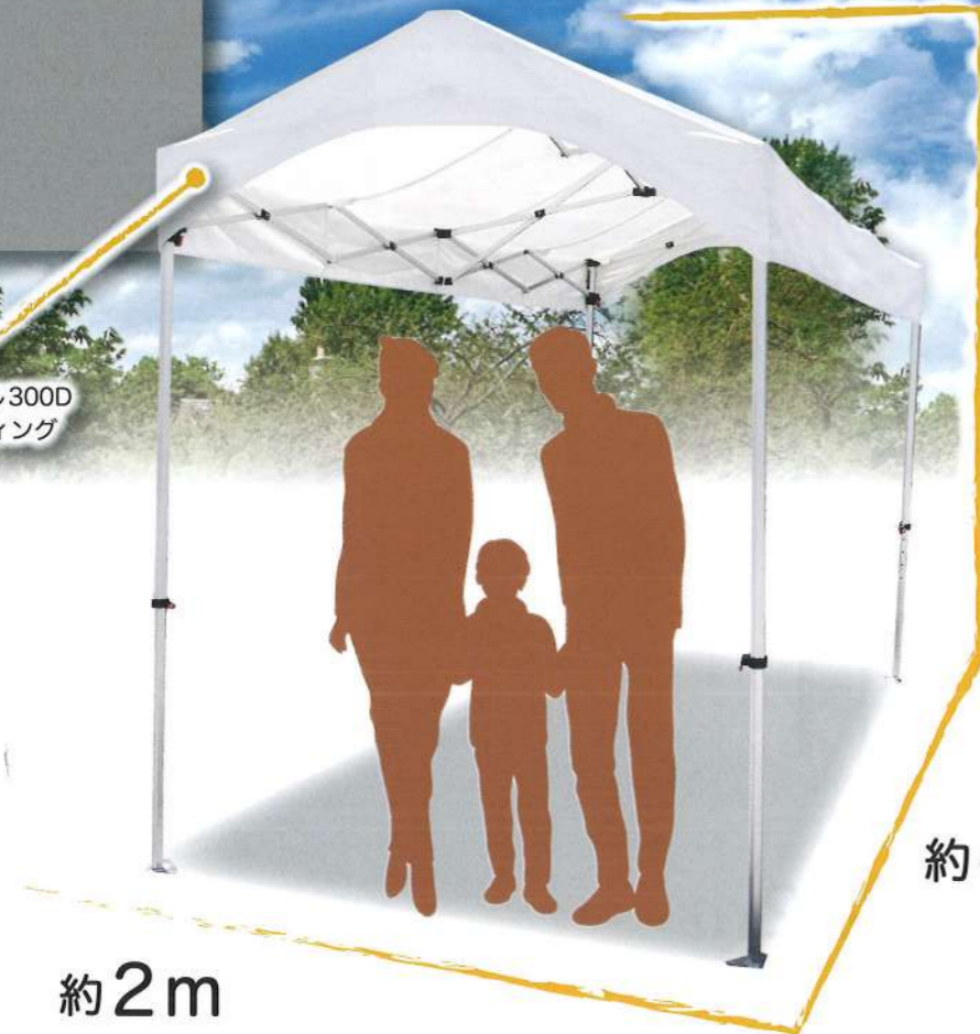
フレーム・天幕 詳細寸法 2m×4.2m
